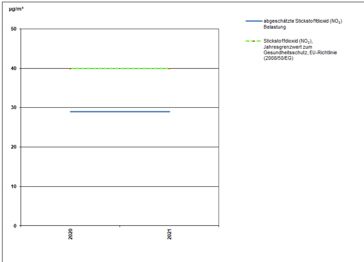
Abbildung 1: Verlauf der absoluten Jahresmittelwerte in \mu\text{g}/\text{m}^3 für NO 2 am MP627
