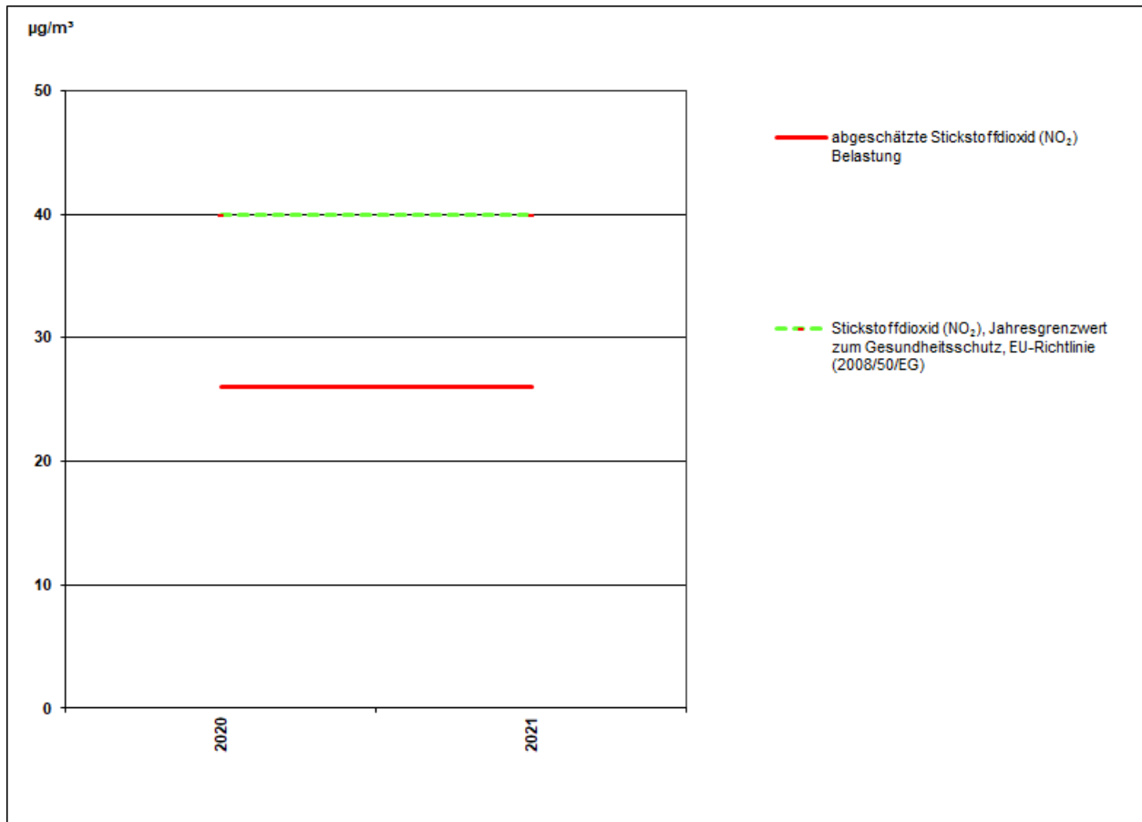
Abbildung 1: Verlauf der absoluten Jahresmittelwerte in \mu\text{g}/\text{m}^3 für \text{NO}_2 am MP623
