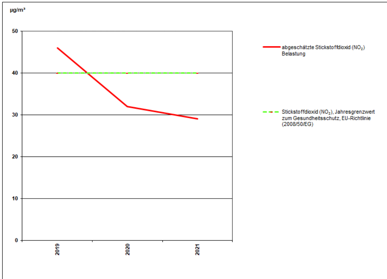
Abbildung 1: Verlauf der absoluten Jahresmittelwerte in µg/m³ für NO 2 am MP613
