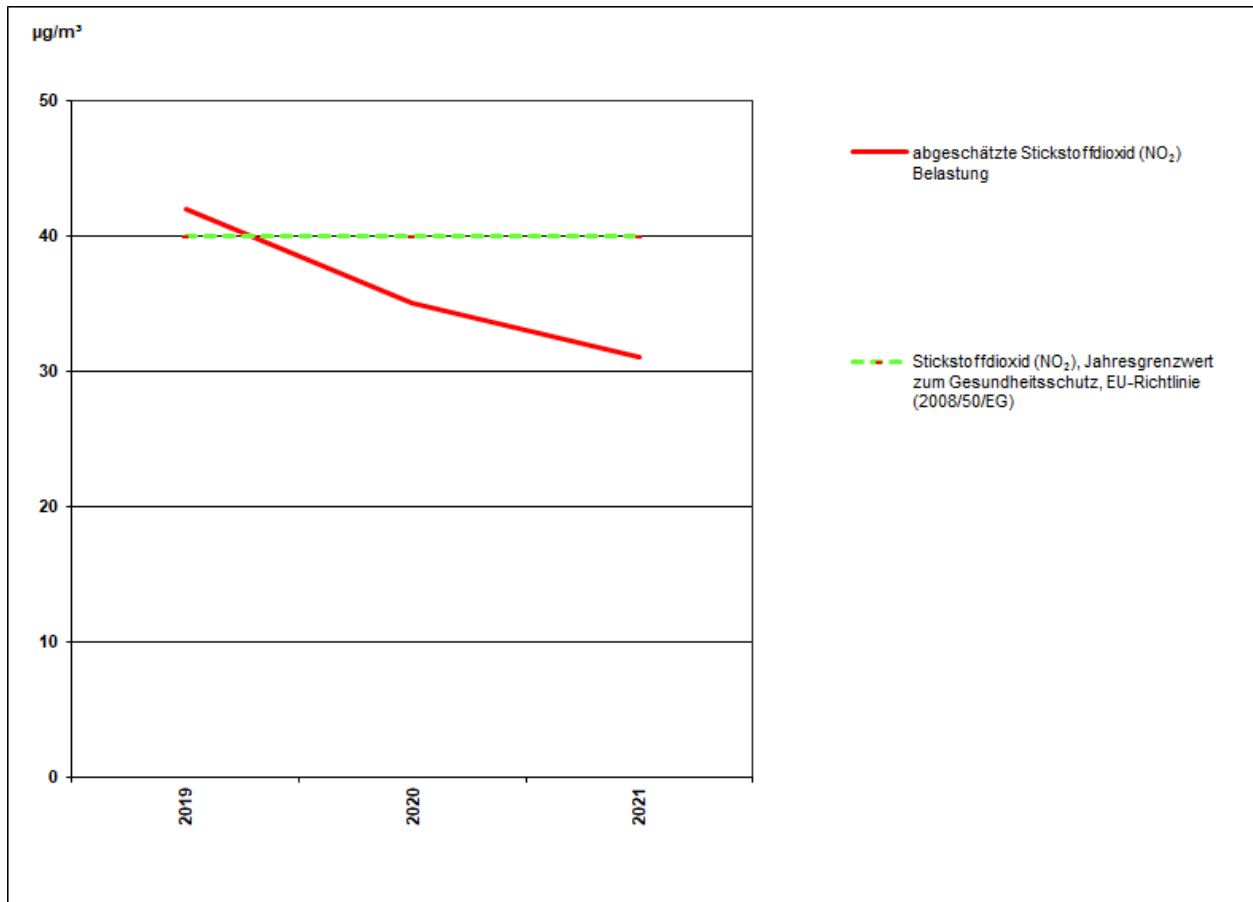
Abbildung 1: Verlauf der absoluten Jahresmittelwerte in µg/m³ für NO 2 am MP610
