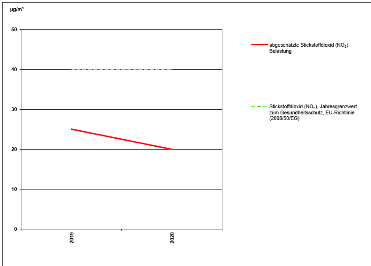
Abbildung 1: Verlauf der absoluten Jahresmittelwerte in µg/m 3 für NO 2 am MP606
