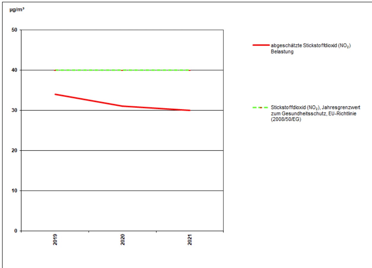
Abbildung 1: Verlauf der absoluten Jahresmittelwerte in µg/m³ für NO 2 am MP603
