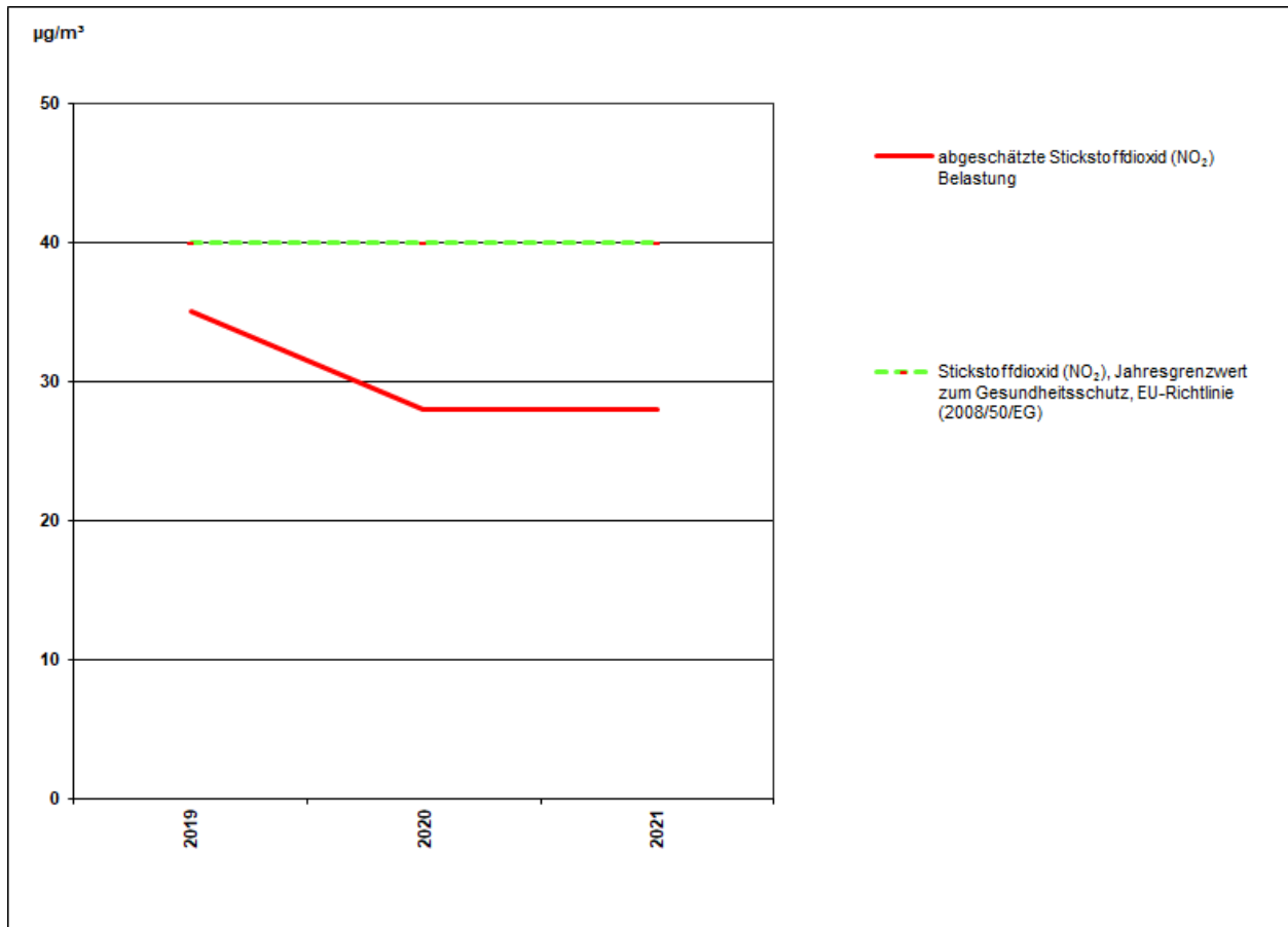
Abbildung 1: Verlauf der absoluten Jahresmittelwerte in \mu\text{g}/\text{m}^3 für NO 2 am MP602
