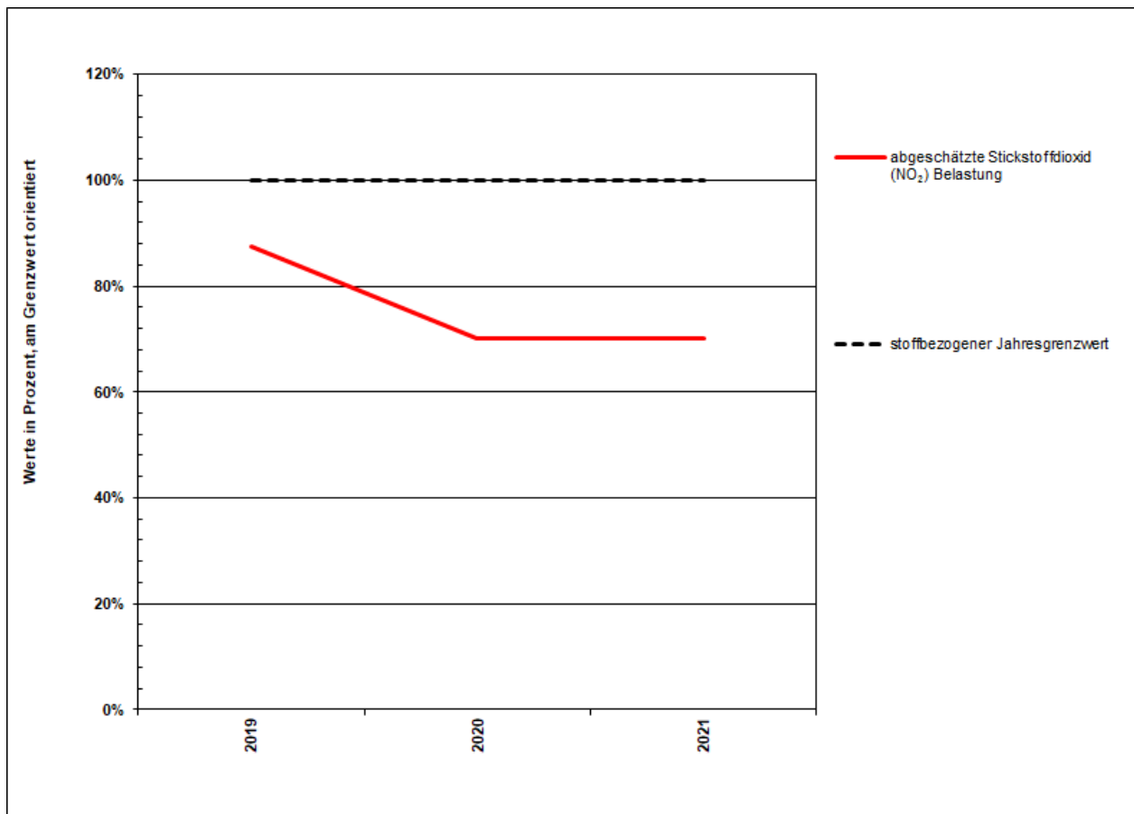
Abbildung 2: Prozentuale Entwicklung der Jahresmittelwerte für NO 2 am MP602
