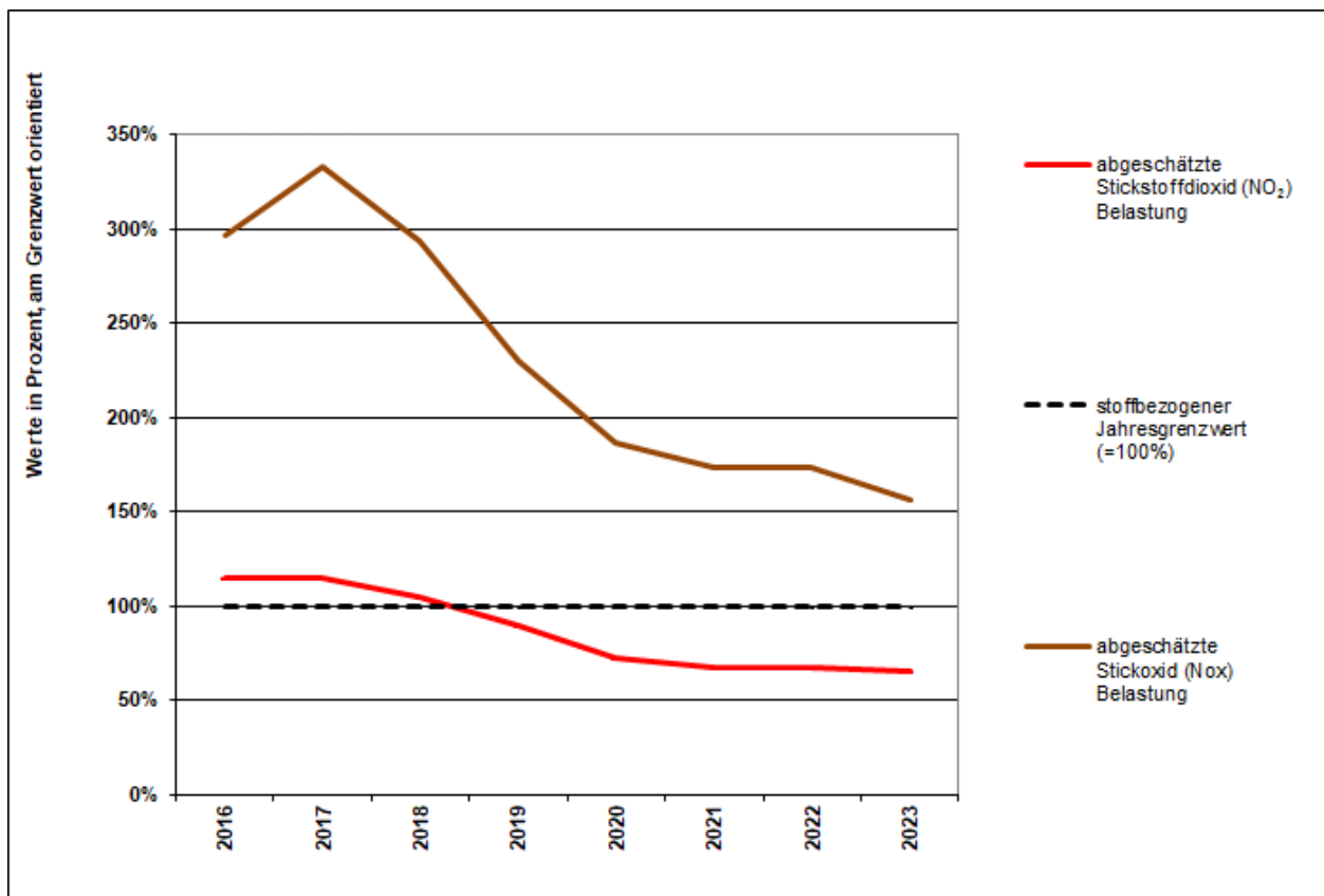
Abbildung 2: Prozentuale Entwicklung der Jahresmittelwerte für NO 2 und NO x am MP582
