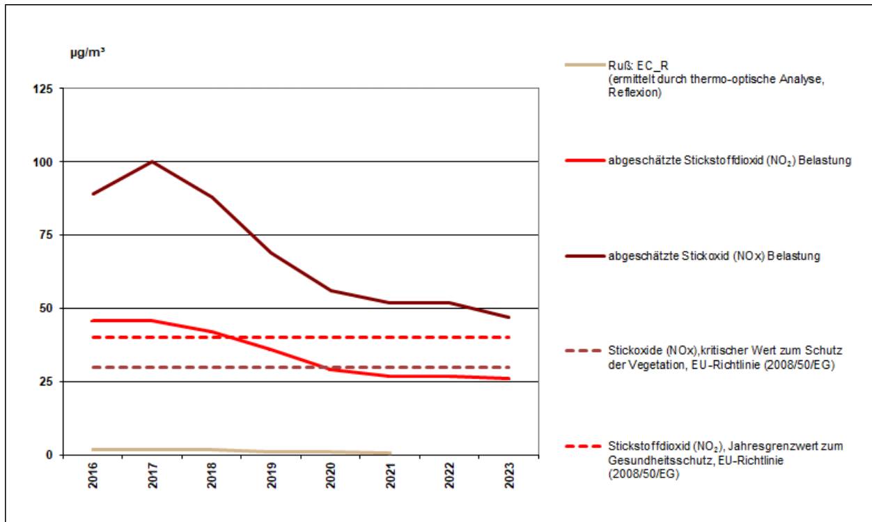
Abbildung 1: Verlauf der absoluten Jahresmittelwerte in µg/m³ für NO 2 , NO x und Ruß am MP582
