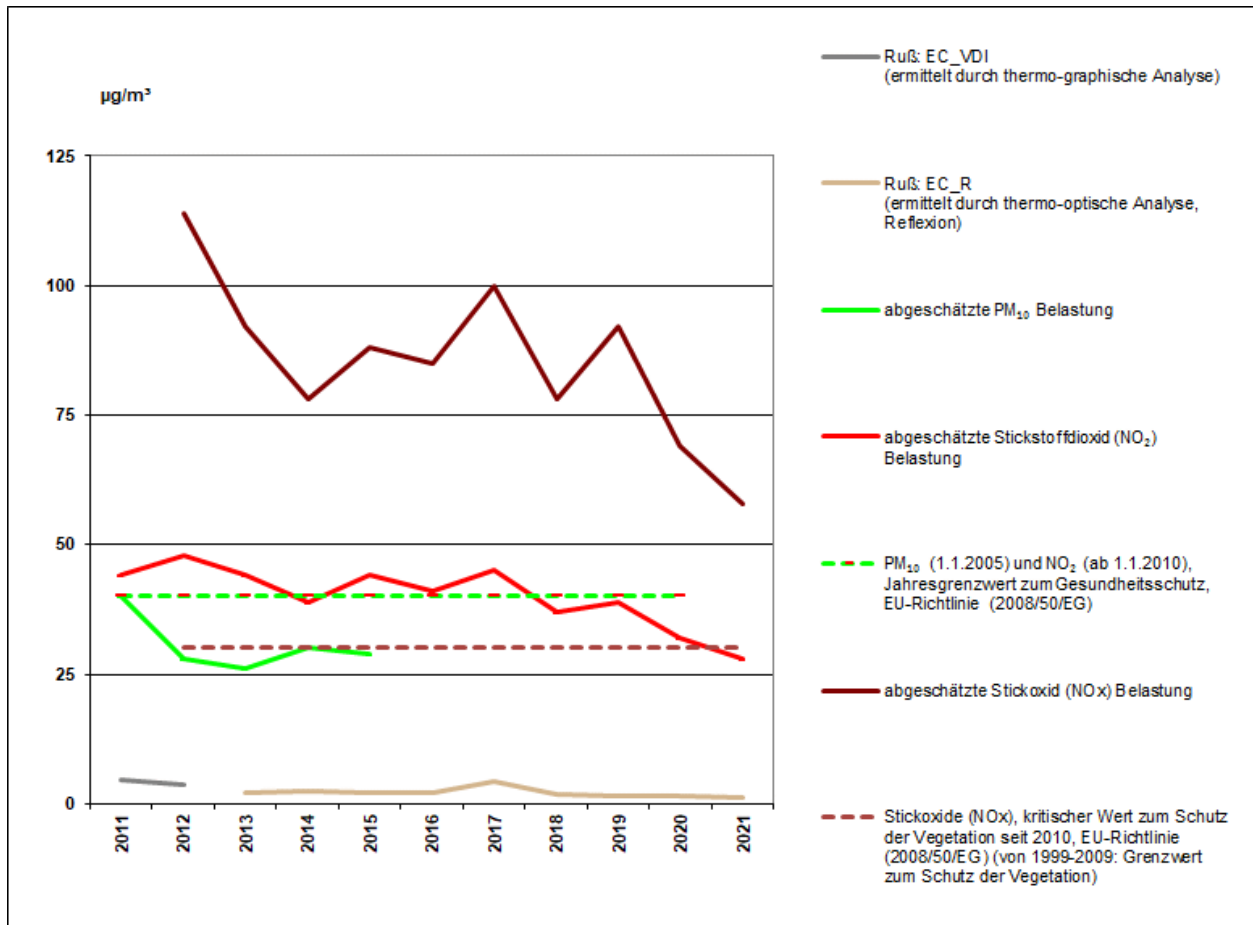
Abbildung 1: Verlauf der absoluten Jahresmittelwerte in µg/m³ für NO 2 , NO x , Ruß und PM 10 am MP581
