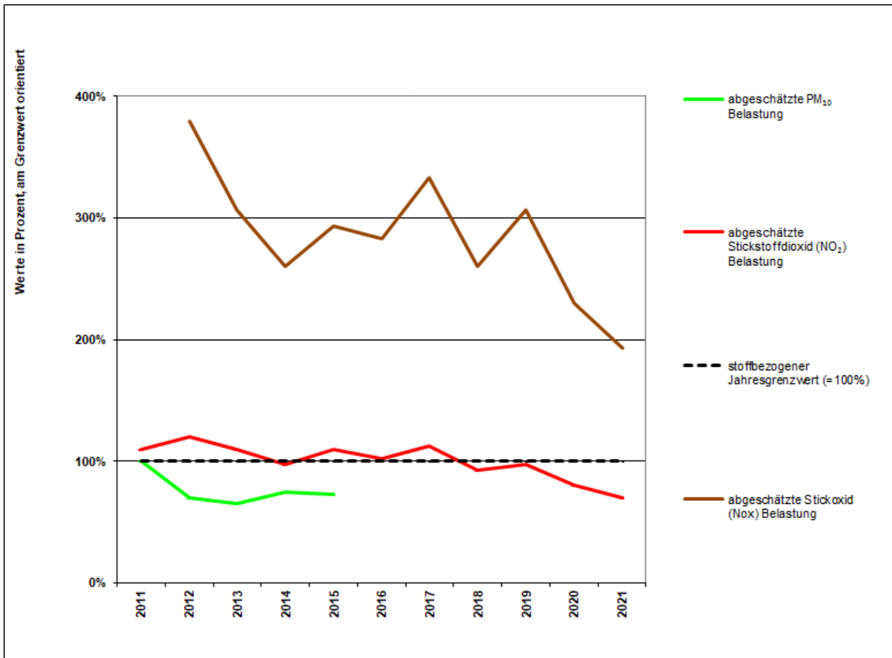
Abbildung 2: Prozentuale Entwicklung der Jahresmittelwerte für NO 2 , NO x und PM 10 am MP581
