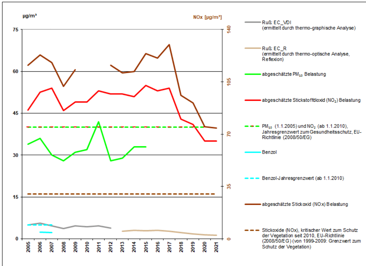
Abbildung 1: Verlauf der absoluten Jahresmittelwerte in \mu\text{g}/\text{m}^3 für \text{NO}_2 , \text{NO}_x , Ruß, \text{PM}_{10} und Benzol am MP573
