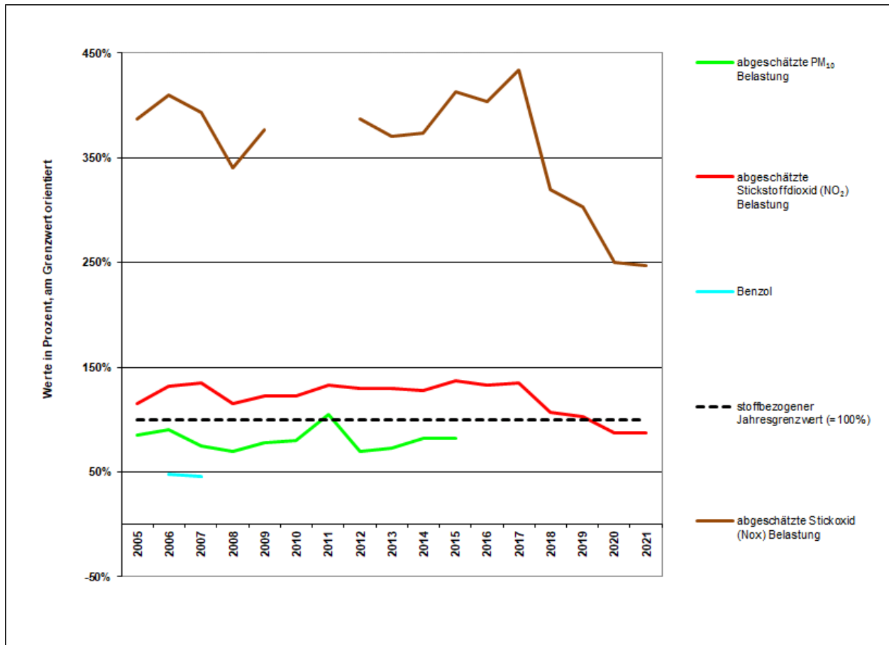
Abbildung 2: Prozentuale Entwicklung der Jahresmittelwerte für NO_2 , NO_x , PM_{10} und Benzol am MP573
