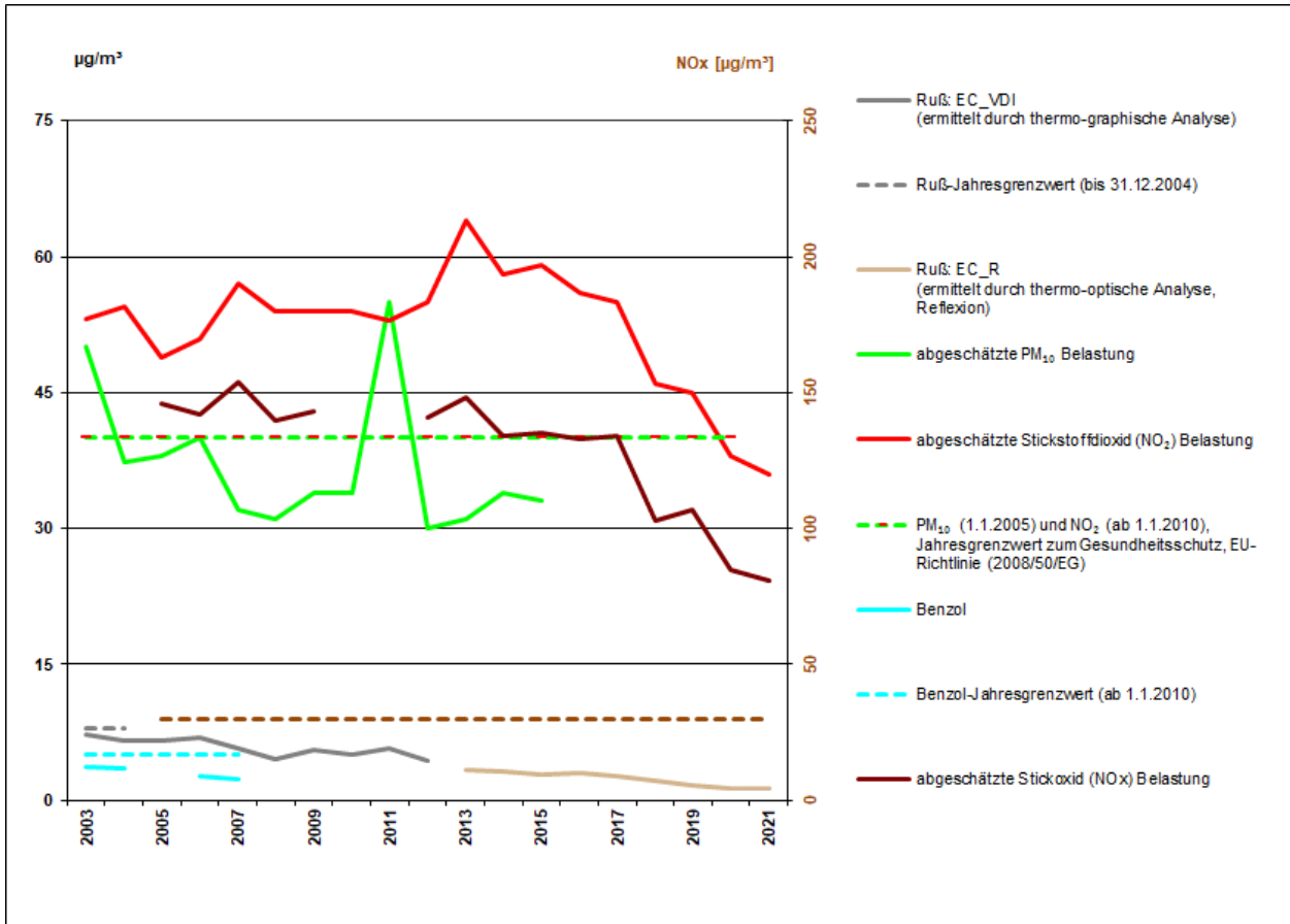
Abbildung 1: Verlauf der absoluten Jahresmittelwerte in \mu\text{g}/\text{m}^3 für NO 2 , NO x , Ruß, PM 10 und Benzol am MP555
