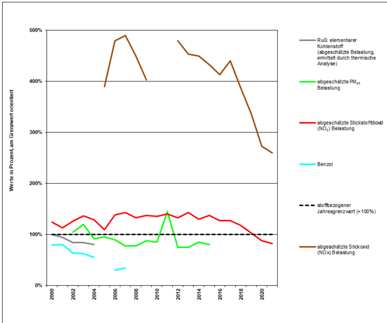
Abbildung 2: Prozentuale Entwicklung der Jahresmittelwerte für NO 2 , NO x , Ruß, PM 10 und Benzol am MP547
