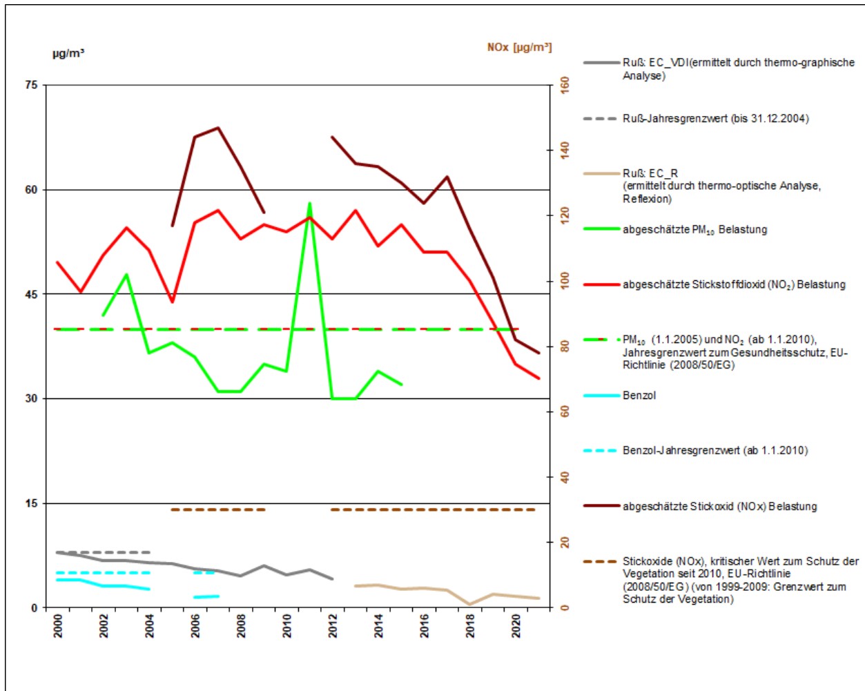
Abbildung 1: Verlauf der absoluten Jahresmittelwerte in \mu\text{g}/\text{m}^3 für \text{NO}_2 , \text{NO}_x , \text{Ru}\ddot{\text{B}} , \text{PM}_{10} und Benzol am MP547
