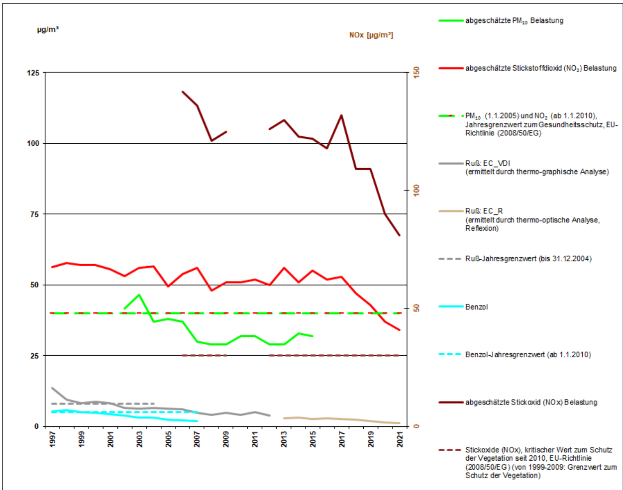
Abbildung 1: Verlauf der absoluten Jahresmittelwerte in µg/m 3 für NO 2 , NO x , Ruß, PM 10 und Benzol am MP514
