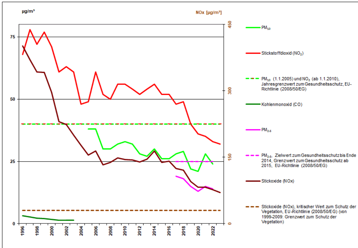
Abbildung 1: Verlauf der absoluten Jahresmittelwerte in µg/m³ für NO 2 , NO x , PM 10 , PM 2,5 und CO am MC143
