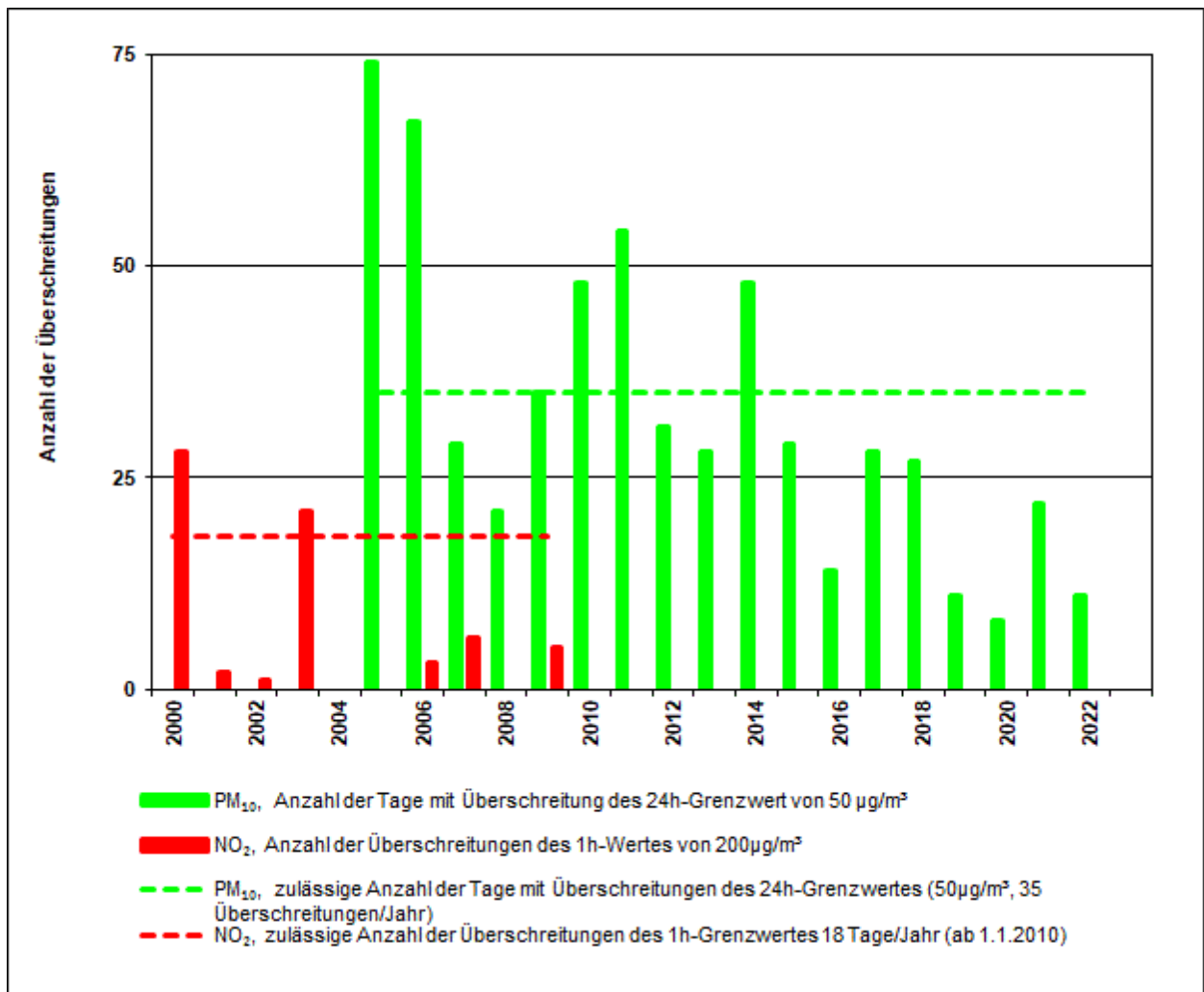
Abbildung 3: Anzahl der Überschreitungen des PM 10 -Tagesmittelwertes von 50 µg/m³ bzw. des NO 2 -Stundenwertes von 200 µg/m³ am MC143
