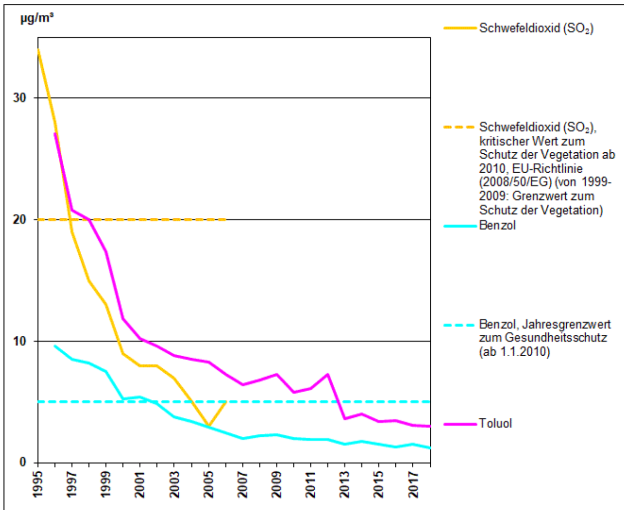
Abbildung 5: Verlauf der absoluten Jahresmittelwerte in µg/m³ für Schwefeldioxid (SO 2 ), Benzol und Toluol am MC117
