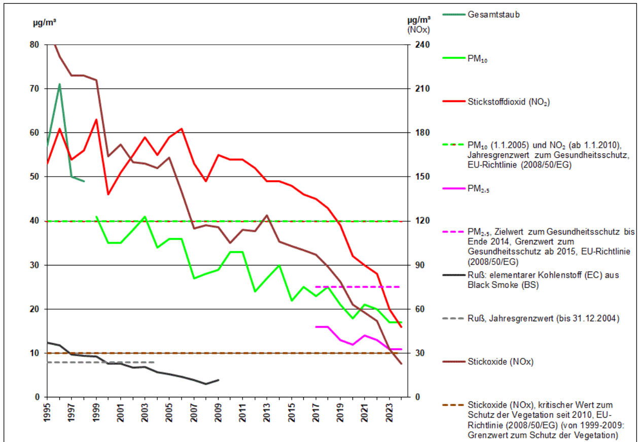
Abbildung 1: Verlauf der absoluten Jahresmittelwerte in \mu\text{g}/\text{m}^3 für \text{NO}_2 , \text{NO}_x , Gesamtstaub, \text{PM}_{10} , \text{PM}_{2,5} und Ruß am MC117
