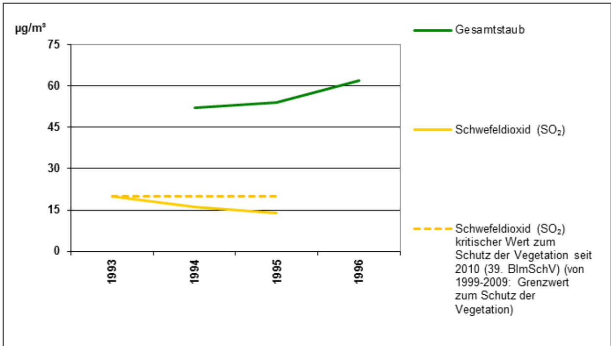
Abbildung 1: Verlauf der absoluten Jahresmittelwerte in µg/m 3 für Gesamtstaub und Schwefeldioxid (SO 2 ) am MC084
