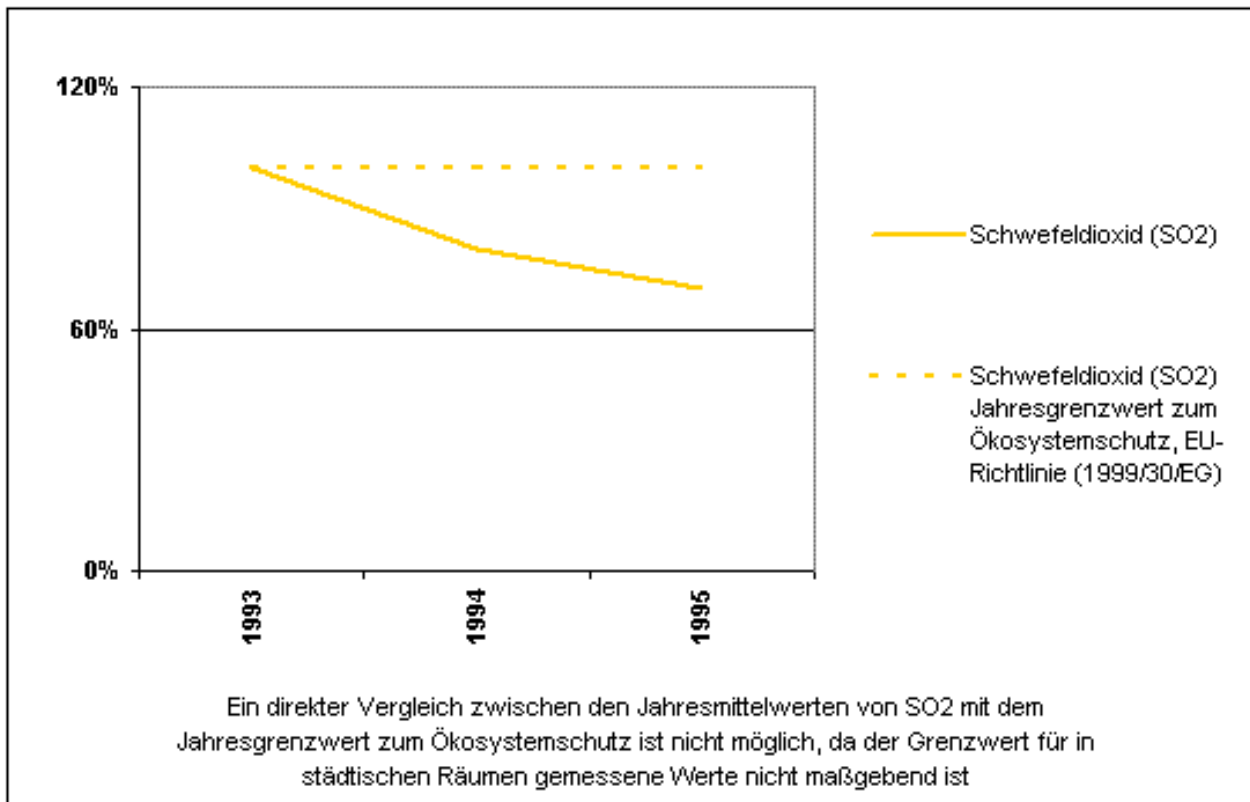
Abbildung 2: Prozentuale Entwicklung der Jahresmittelwerte für Schwefeldioxid (SO 2 ) am MC084
